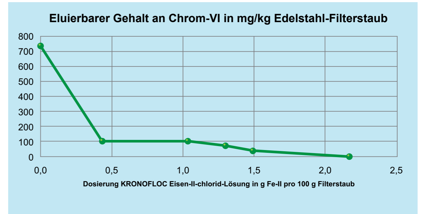
Abb. 6: Eluierbarer Gehalt an Chrom-VI in Edelstahlwerks-Filterstaub bei verschiedenen Dosierungen von Eisen-II-chlorid-Lösung KRONOFLOC
